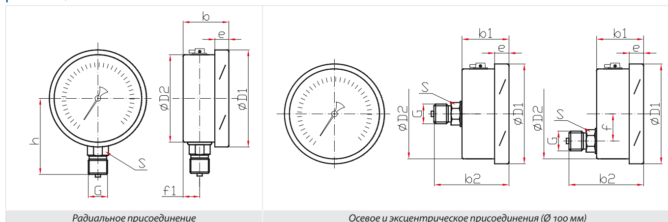
Радиальное присоединение
