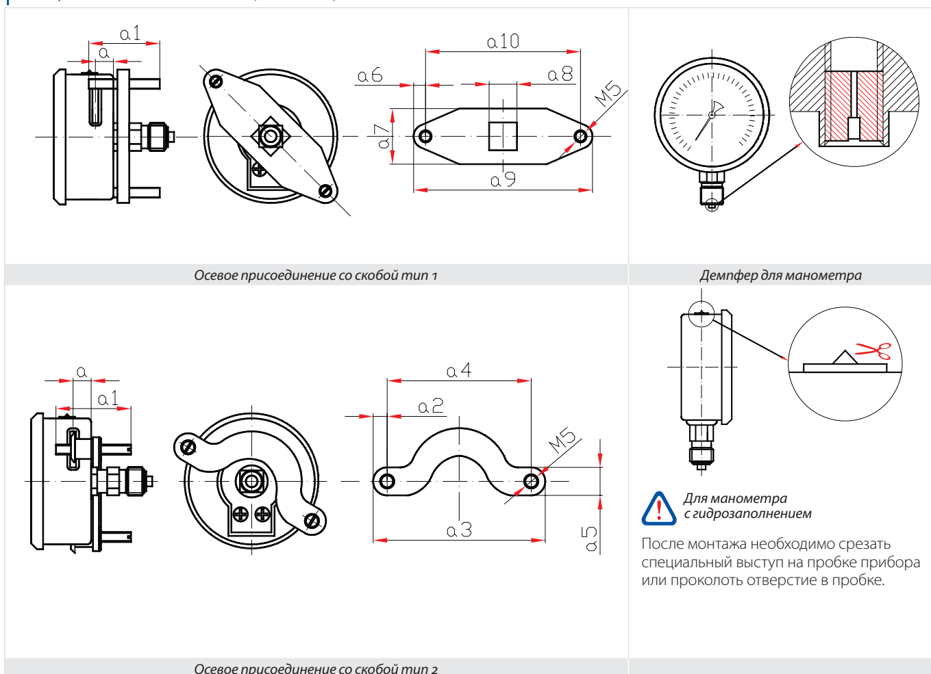
Основные размеры (мм)
